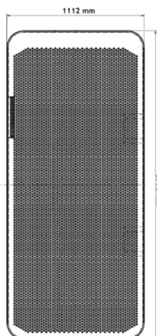
1,6 m 2 PP-plate Diaphragm
