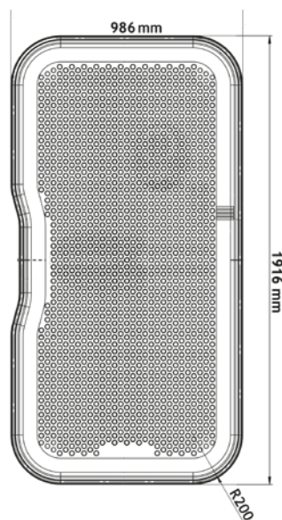
1,6 m 2 PP-plate Diaphragm
